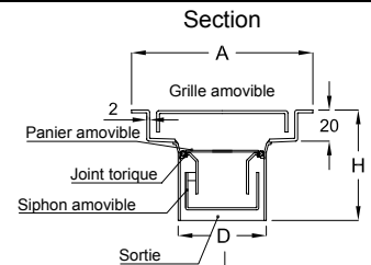
Inoxsystem® IDrain 3068 - Siphon avec grille standard et fente périmétrale - carré bords visibles - sortie horizontale - siphon et panier amovibles
